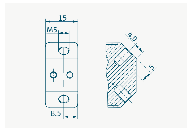
流体安装尺寸，单位为 mm
